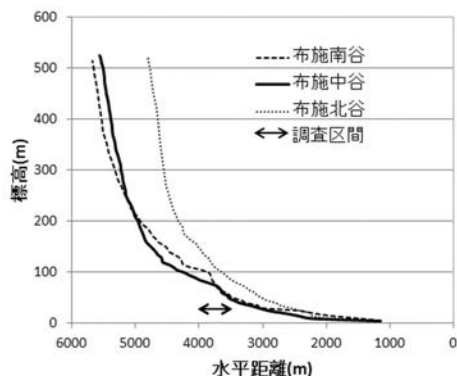
図3 春日川3支川の河床縦断形
