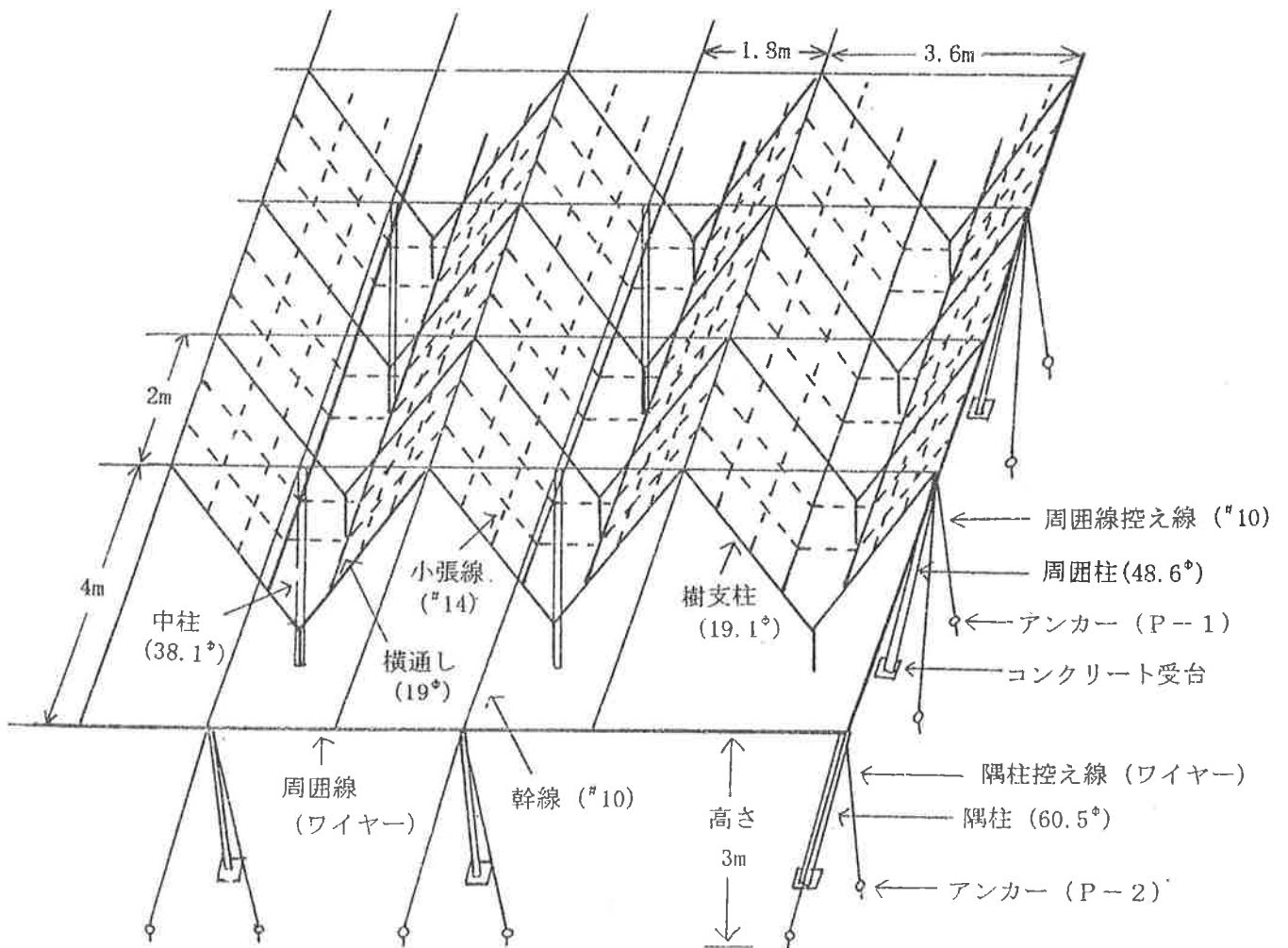
第2図 リンゴY字形棚 (ネット兼用棚)
