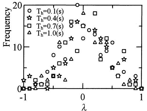
図-3 \lambda の度数分布 [ T_v=0.2(s) の場合]
