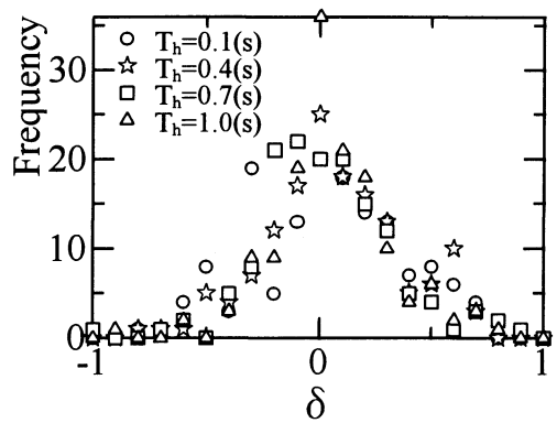
図-2 \delta の度数分布
